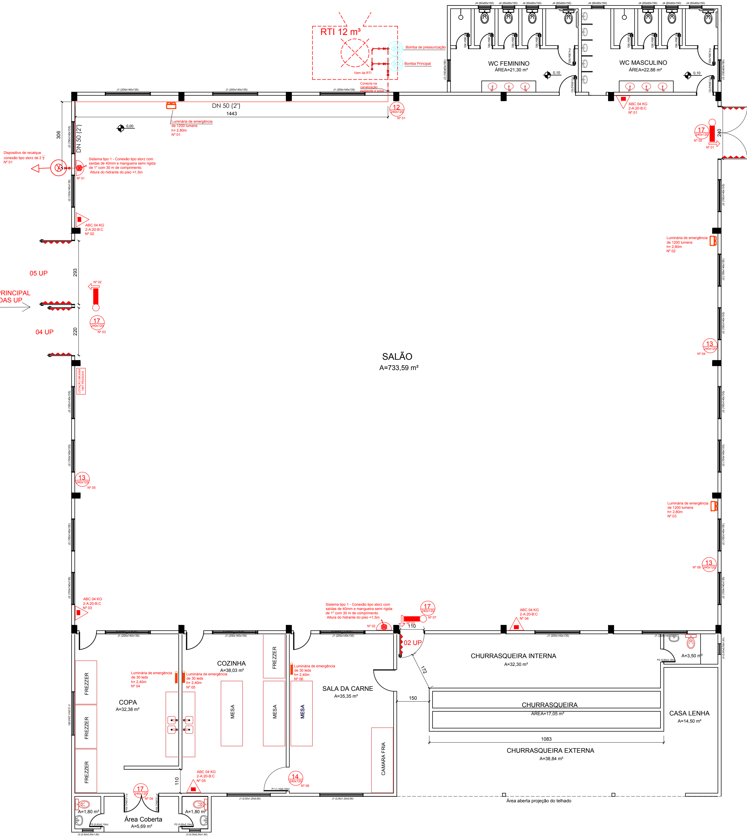
PLANTA BAIXA EDIFICAÇÃO A= 1036,24m²
